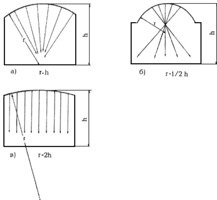
Рисунок 5 - Варианты решения зала с куполом
